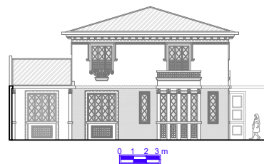
Elevação 02
