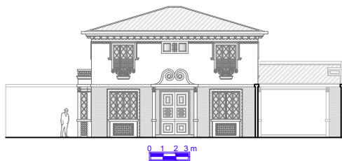
Elevação 01
