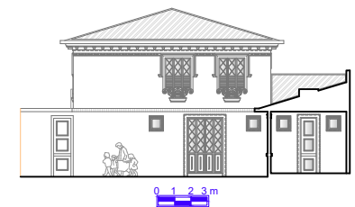
Elevação 04
